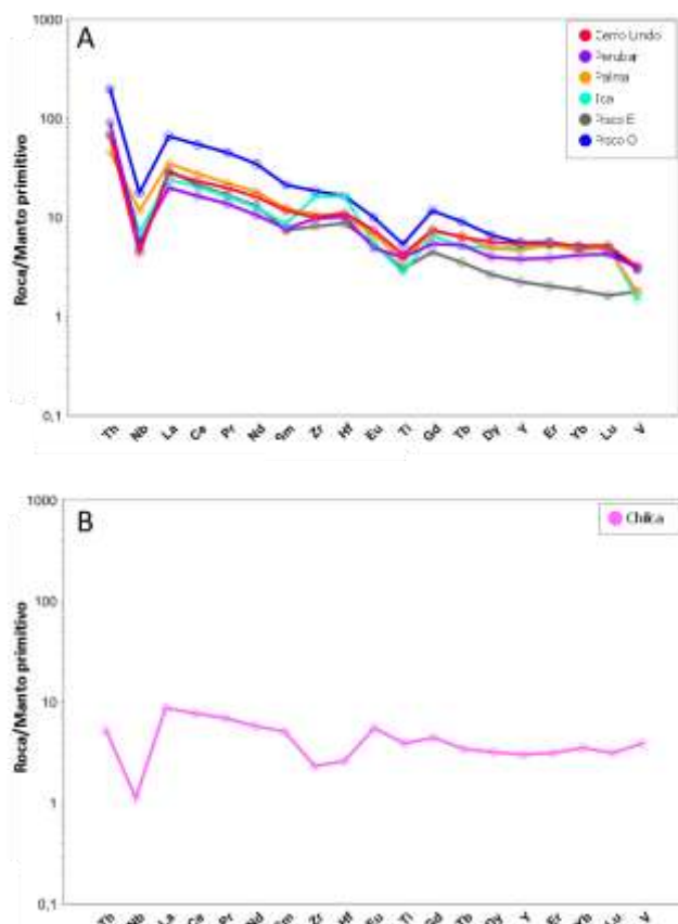
Figura 04. Diagrama tipo spider de los dos tipos de firmas. A. Enriquecimiento de LREE en rocas asociadas a los depósitos VMS. B Relación plana de LREE y HREE en una muestra al NO de la cuenca.
