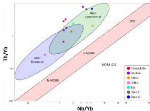
Figura 03. Th/Yb versus Nb/Yb de Pearce (2014).
