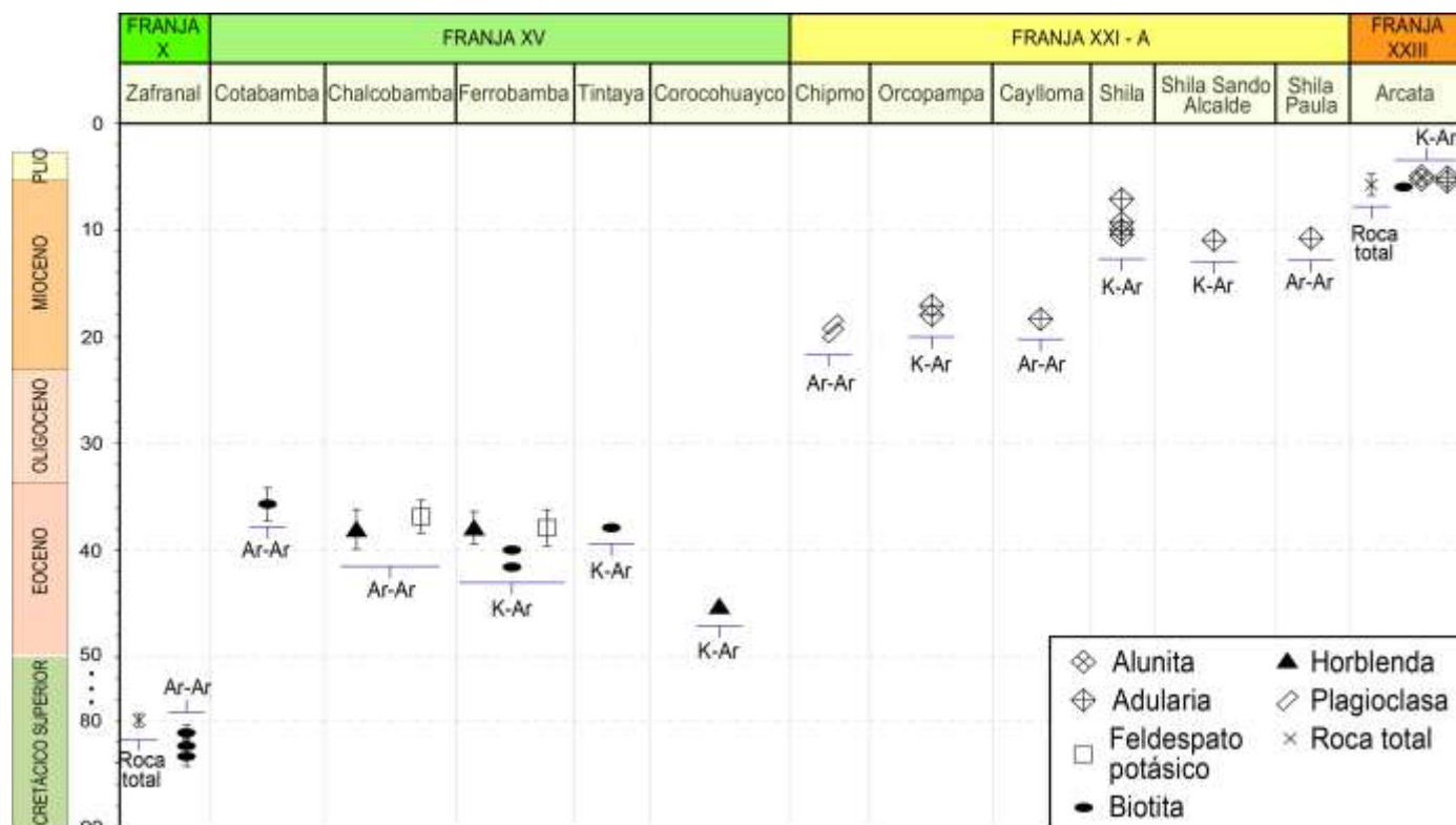
Figura 2. Cuadro resumen de las edades geocronológicas de cristalización, alteración y mineralización de los principales yacimientos de las regiones Cajamarca y La Libertad, según franja metalogénica.
