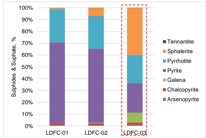
Figura N°6: Mineralogía del compuesto LDFC-03
