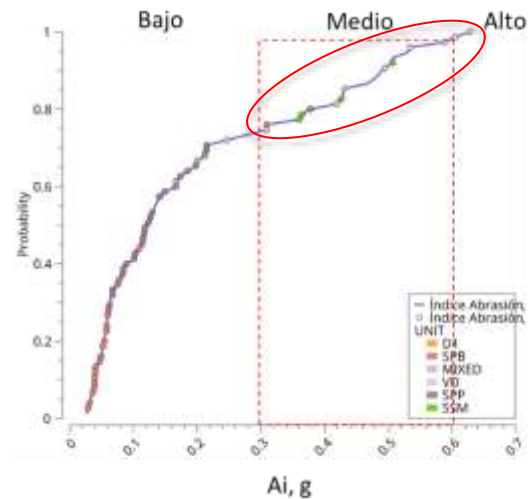
Figura N°4: Índice de abrasión (Ai)
