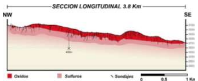
Fig. 5. Sección longitudinal con estados de mineralización en profundidad.
