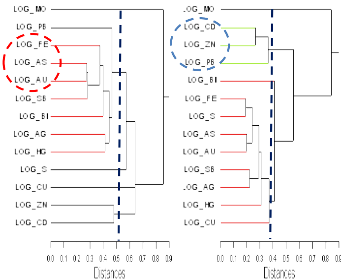
Fig. 4. Agrupación jerárquica Pearson para la zona de Óxidos (izquierda) y Sulfuros (derecha).
