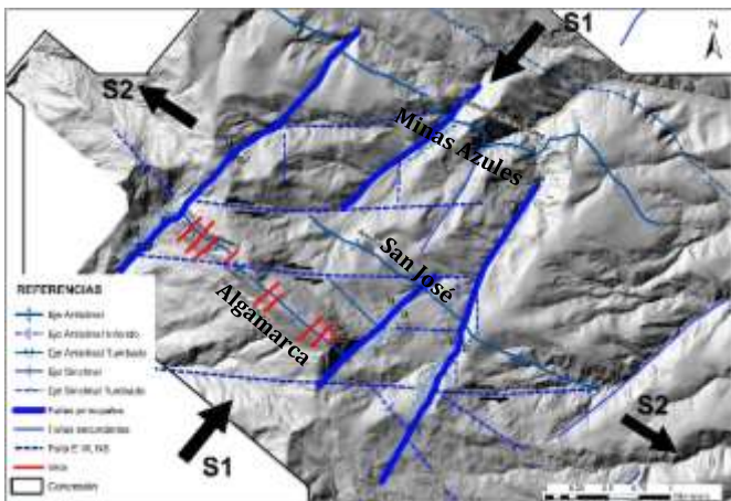
Fig. 1. Un primer evento, causante de las principales estructuras generadas por compresión que controlan la mineralización de las vetas del cerro Algamarca (similar a un arreglo Riedel Sinestral (Transpresivo)).
