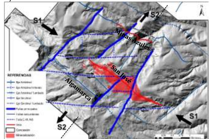
Fig. 2. Un segundo evento, causante de las principales estructuras mineralizadas, generadas por compresión de tendencia NW-SE que controlan la mineralización de la zona de Shahuindo (similar a un arreglo tipo Riedel, dextral (Transpresivo)).
