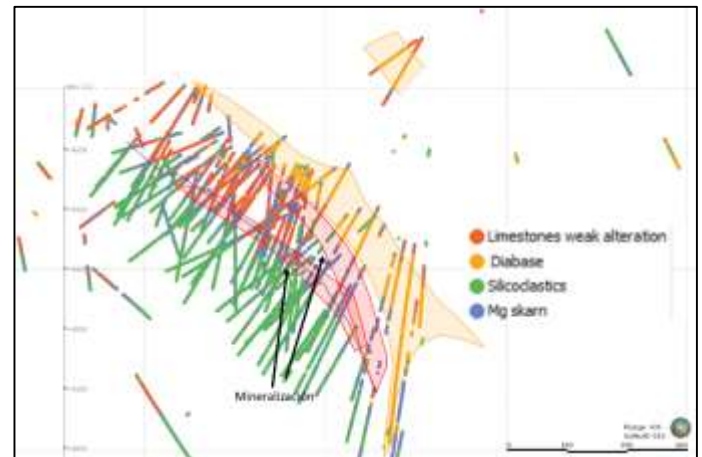
Figura 6. Resultado de la clusterización litológica.
