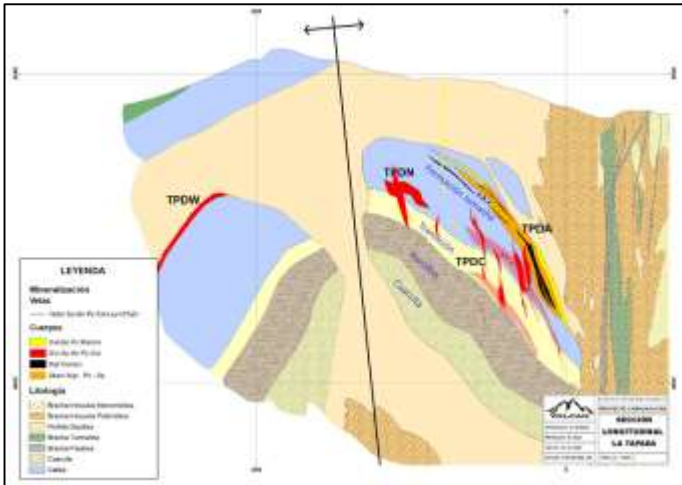
Figura 2. Sección geológica mirando al norte en La Tapada.
