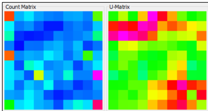
Figura 4. Matrices de conteo (izquierda) y de distancia unificada (derecha).
