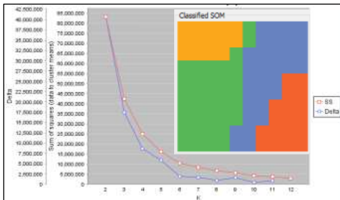
Figura 5. Clasificación SOM por K-means.
