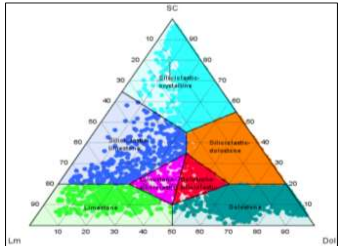
Figura 3. Diagrama para la clasificación de rocas químicas-silicoclásticas según Ordoñez-Calderón et al. (2017), usando datos de La Tapada.
